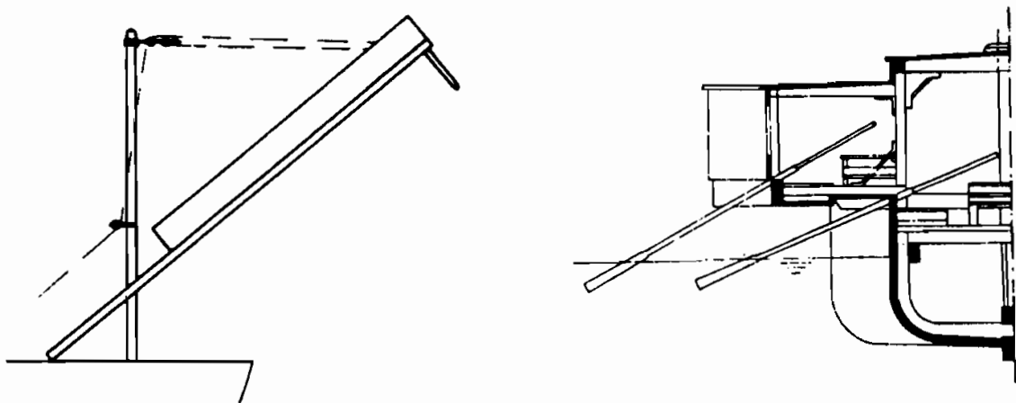
شکل ۱.۱۳ پل‌های چوبی مورد استفاده رومیان در جنگ اول پونیک
