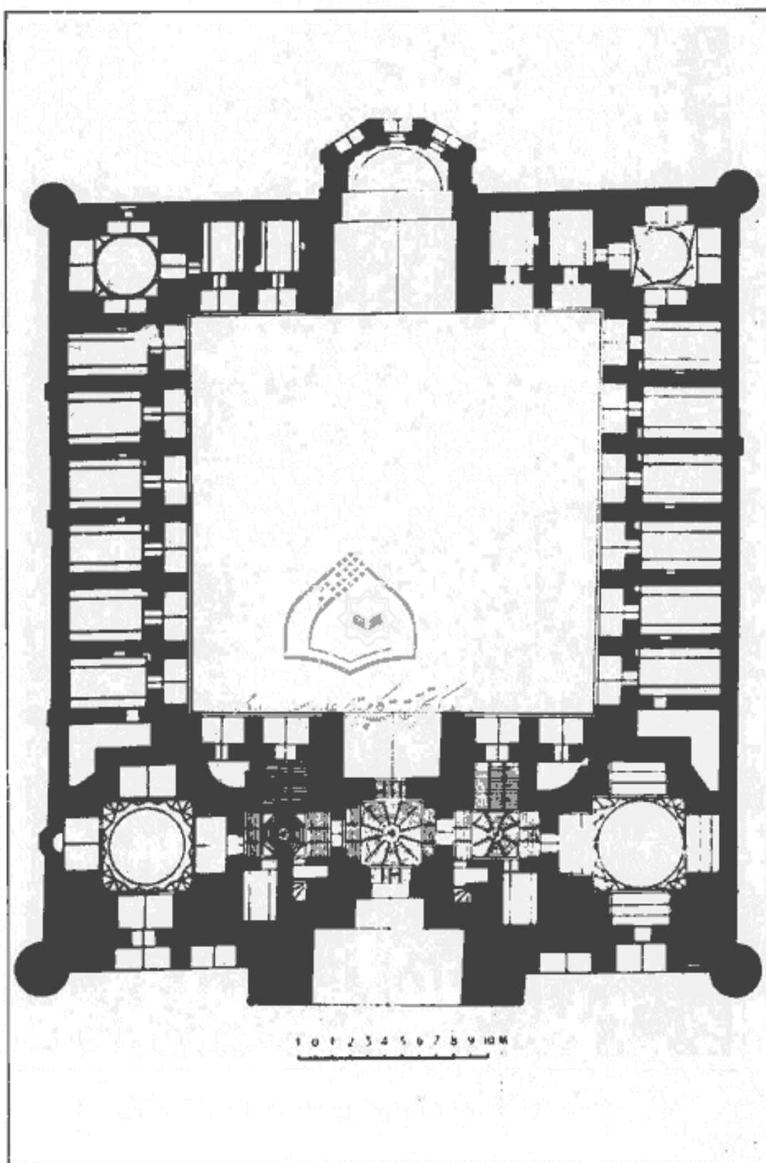
۸۱- نقشه (پلان) مدرسه الغ بیك بخارا.
