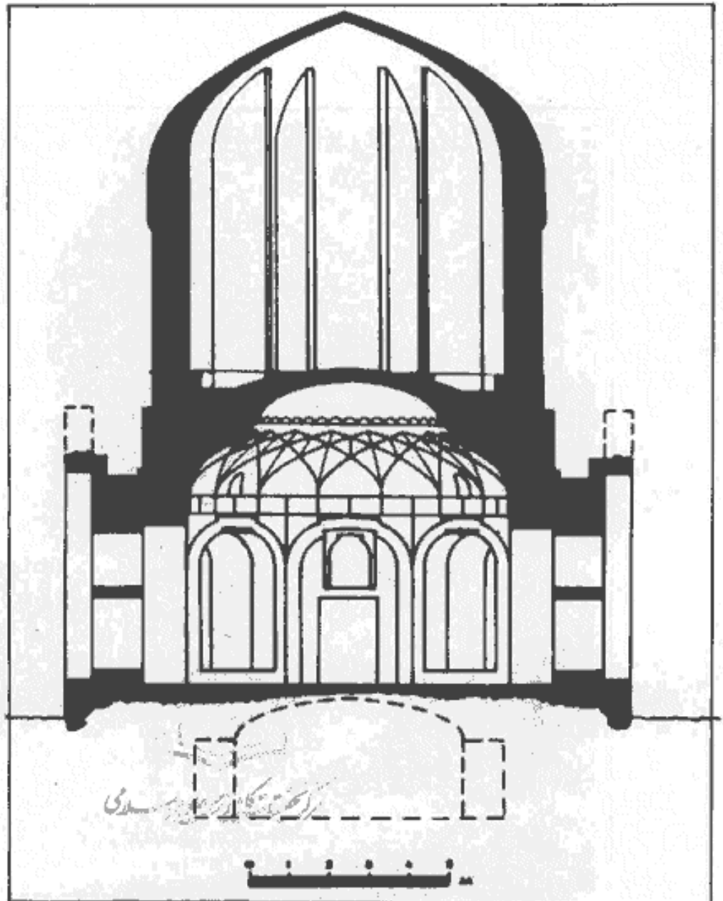
۵۸- مقطع عمودی مصلی گوهرشاد، هرات.
