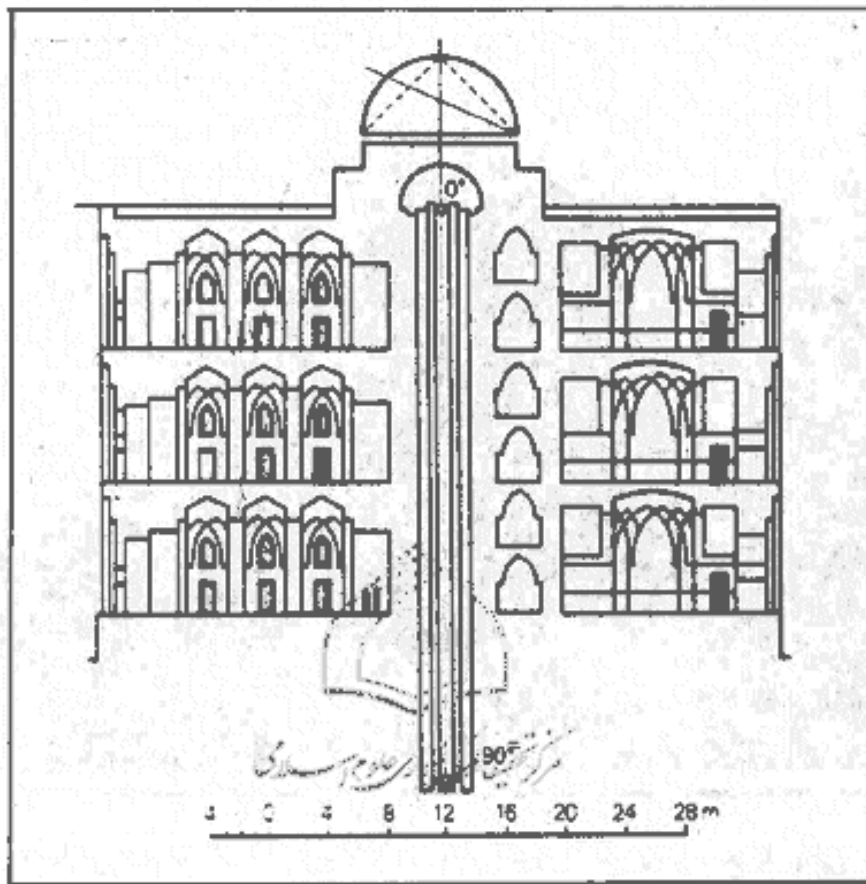
۷۵- مقطع عمودی از رصدخانه السغریک (بر اساس منابع تاریخی و کاوشهای باستان‌شناسی).
