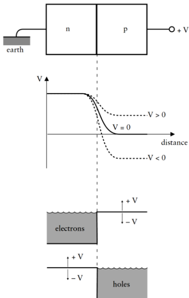
شکل ۳-۹: گرِهی که از اتصال دو قطعه سیلیکون نوع n و نوع p تشکیل شده است.
