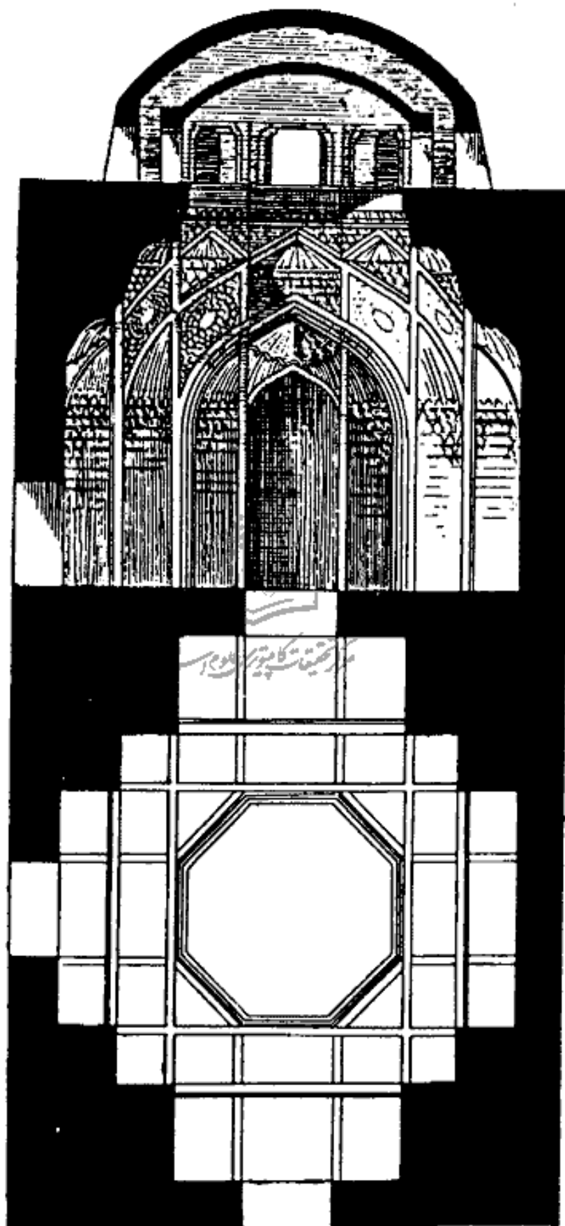
تصویر ۴. خرجرد، مدرسه، پلان و بخشی از گنبدخانه شرقی
